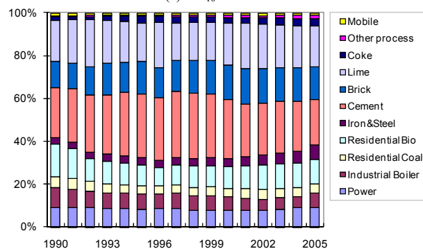
(d) TSP emissions
