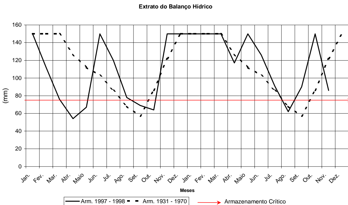
Figura 1 – Valores do armazenamento mensal (ARM) ocorridos no período de jan 1997/nov 1998 e 1931- 1970 (normal), segundo cálculo do balanço hídrico (Tornthwaite & Mather, 1955) – 300 mm, para o município de Limeira-SP.
