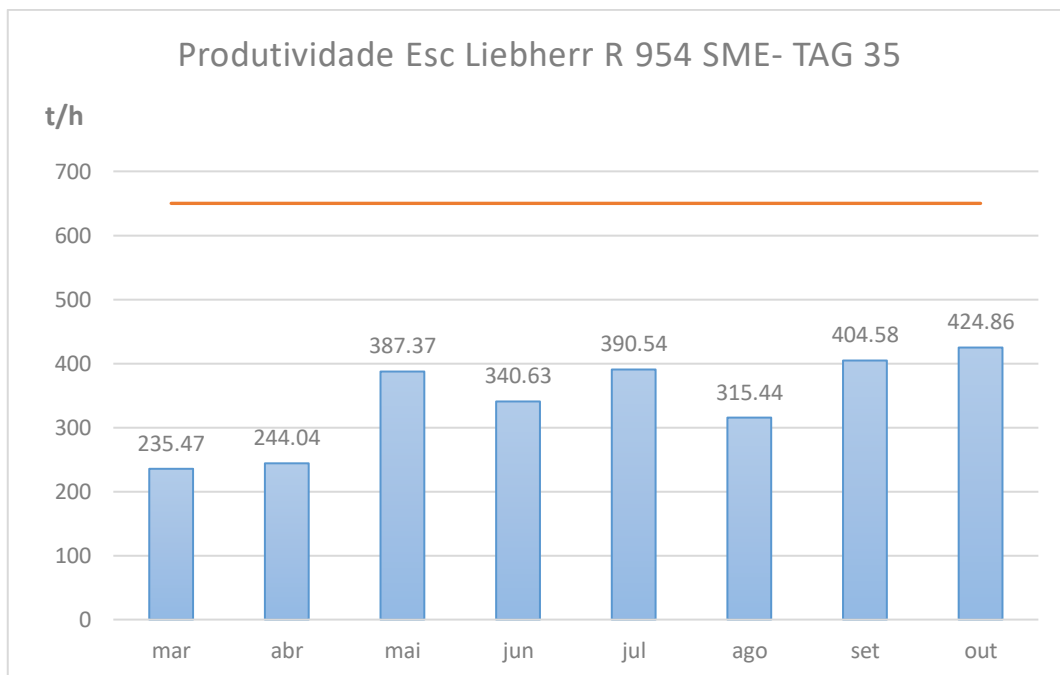
Figura 30 Produtividade escavadeira TAG 35
