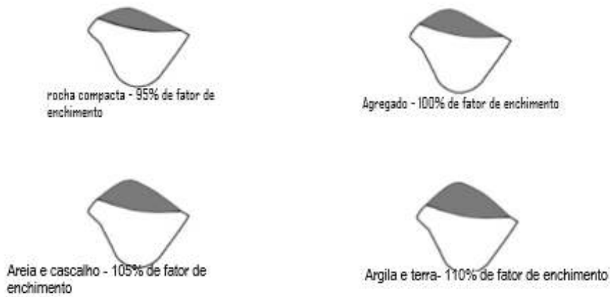
Figura 15 Fator de enchimento segundo material de carregamento
