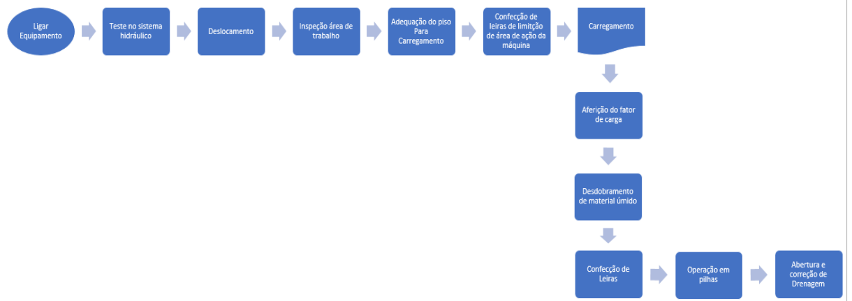
Figura 34: Mapa de processos carregadeira
