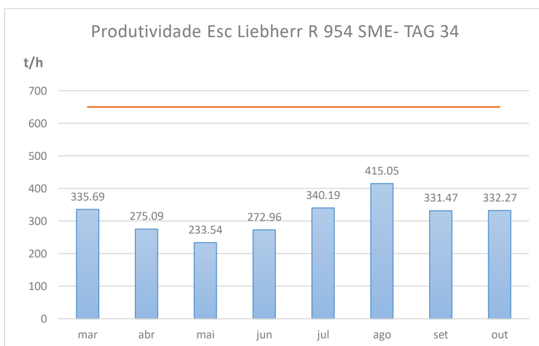
Figura 29 Produtividade escavadeira TAG 34
