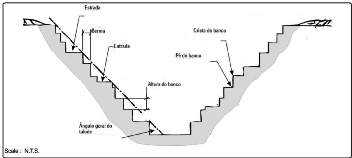
Figura 2 Elementos de uma lavra por bancadas.
