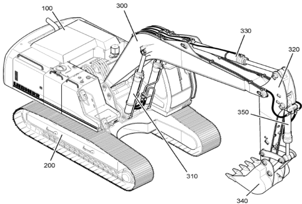
Figura 12 Principais componentes da escavadeira R 954 C SME Liebherr
