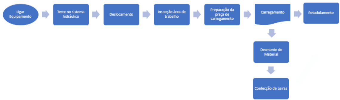
Figura 33 Mapa de processo Escavadeiras
