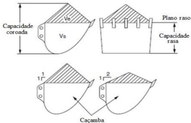
Figura 14 Volume da caçamba
