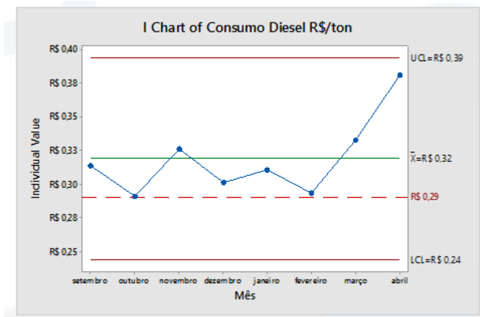
Figura 20 Carta controle inicial do KPI
