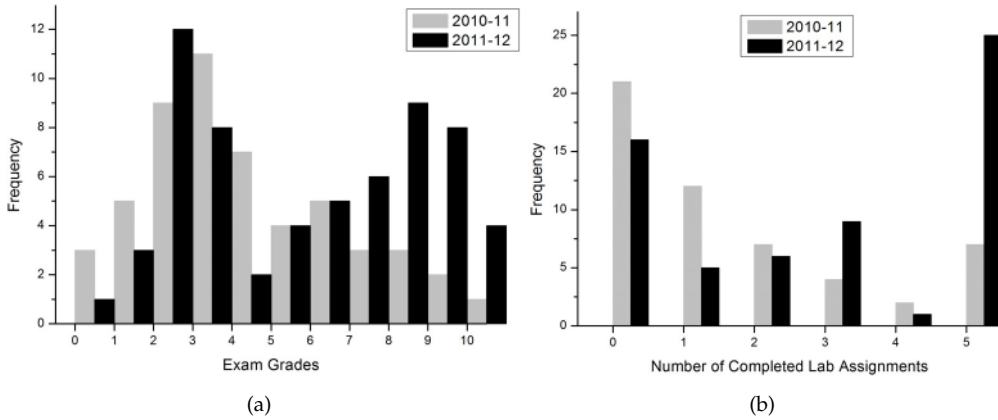
Fig. 10. Dataset Histograms
