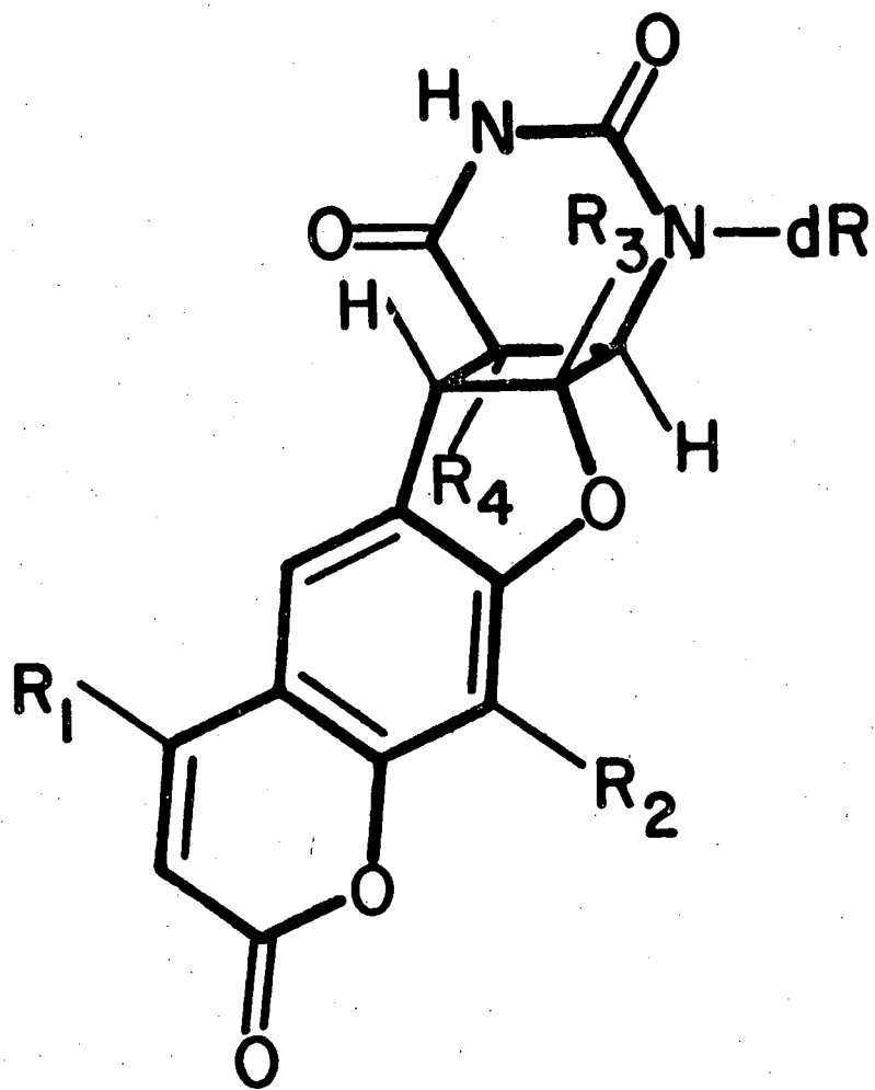
trans-syn-5
