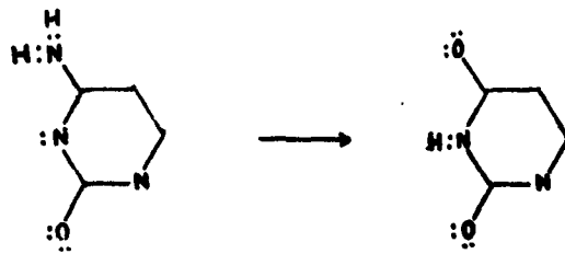
cytosine
