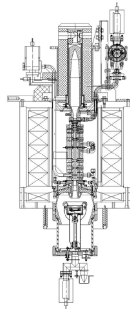
Figure 3: SLAC XL-4 50MW Klystron.
