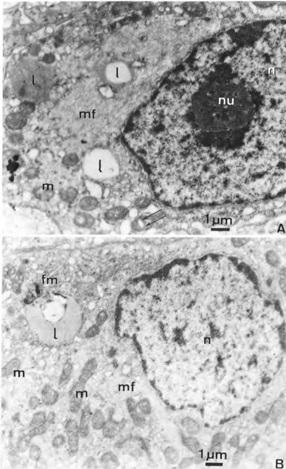
FIGURA 3: A e B - Células de Leydig de burro, mostrando características intermediárias entre as de cavalo e jumento. (l = lipídio; n = núcleo; nu = nucléolo; mf = microfilamentos; m = mitocôndrias; fm = figura mielínica)
