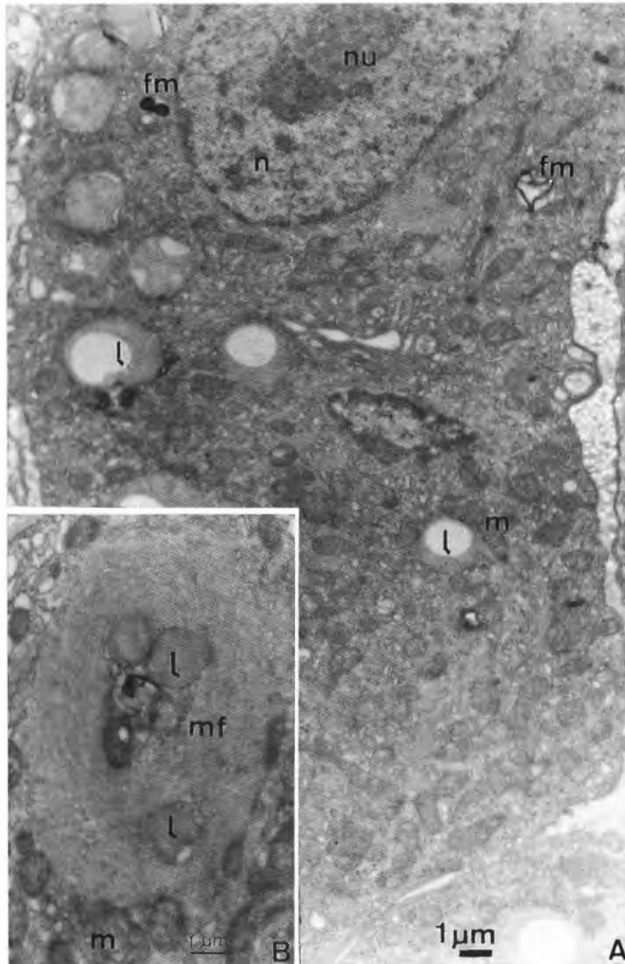
FIGURA 4 - Células de Leydig de burros. A) Aspecto do citoplasma da célula de Leydig mostrando grânulos de lipídio (l). B) Microfilamentos (mf) dispostos com arranjo concêntrico. (fm = figura mielínica; n = núcleo; nu = nucléolo; m = mitocôndria)
