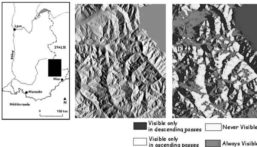
FIG. 1. – Simulation of the geometrical visibility for ERS radar images over the French South Alps. a) The black box corresponds to the extension of the study area. b) Shaded relief map of the study area. c) Visibility map of the study area. FIG. 1. – Simulation de visibilité pour les images radar ERS sur les Alpes françaises du Sud. a) Extension de la zone d’étude. b) Carte de relief (ombrage) de la zone d’étude. c) Carte de visibilité de la zone d’étude.
