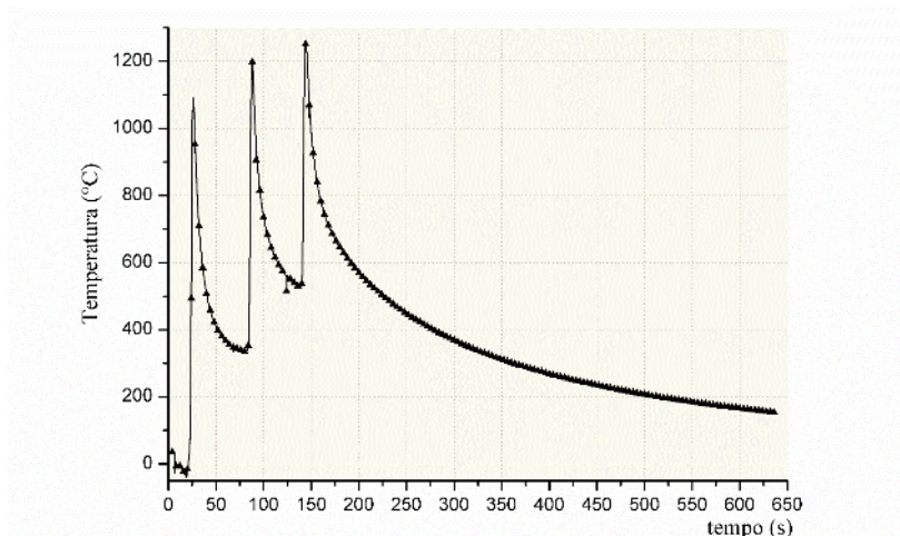
Figura 4. Ciclo térmico de soldagem para a amostra 0-33.
