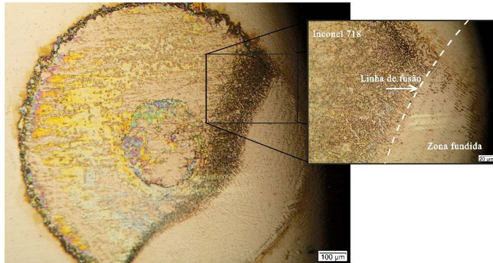
Figura 9. Micrografia da região de interface ZF/Inconel 718 mostrando região de corrosão mais severa na ZTA do Inconel da amostra 0-50. Microscopia ótica. Sem ataque metalográfico.
