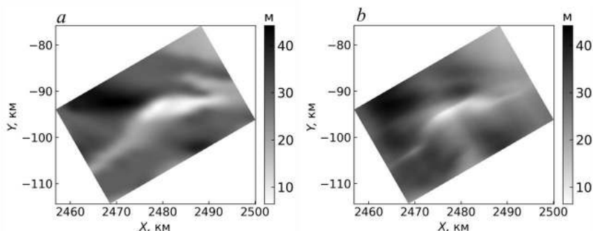
Р и с. 9. Особенность A (см. рис. 5) поля донной топографии ( a ); восстановленная интегрированием (4) глубина в том же районе ( b )
