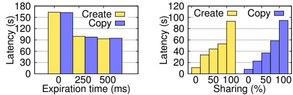
(a) Metadata cache.
