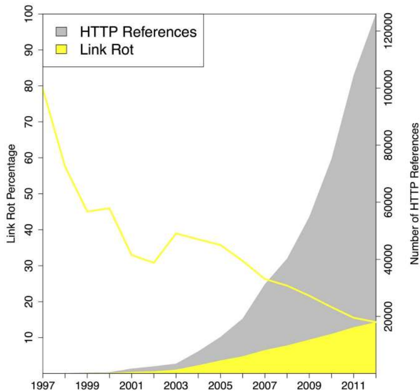
Fig. 12. Link Rot - PMC corpus.
