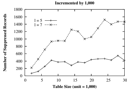
Fig. 10. Suppression
