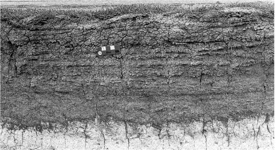
FIG. 9. Manto eólico con estructuras internas parcialmente conservadas. FIG. 9. Aeolian blanket with partially preserved internal structures.
