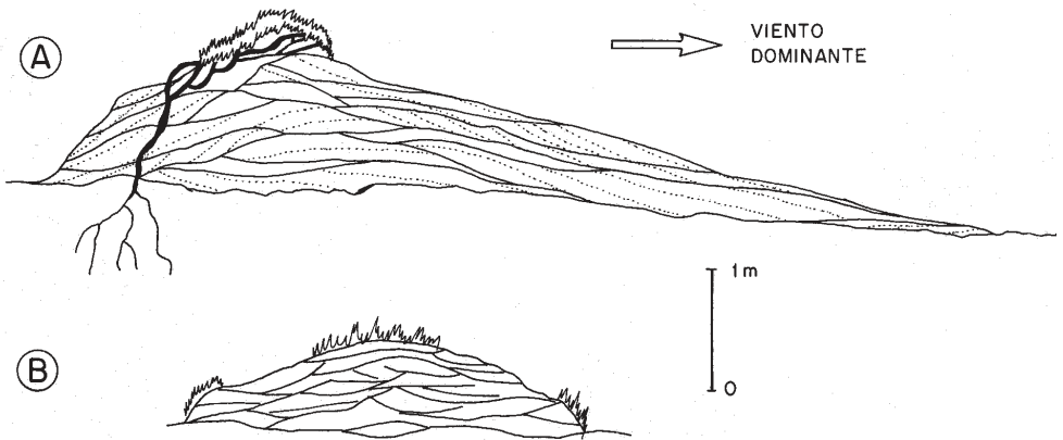
FIG. 5. Estructuras internas de las dunas de arcilla según ejemplos de campo. A. Dunas asimétricas en forma de cometa. B. Dunas hemisféricas.
