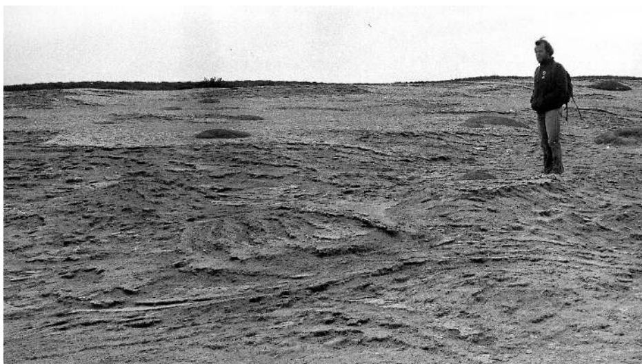
FIG. 6. Estratificación cruzada compleja en un campo de dunas asimétricas.
