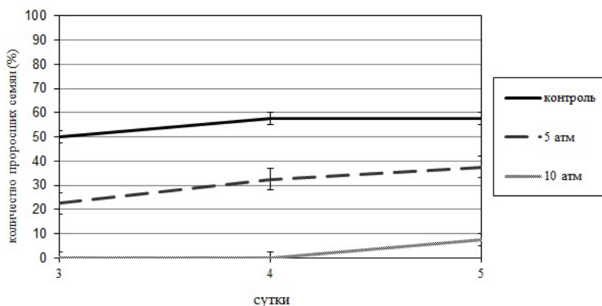
Рис. 4. Динамика прорастания семян T. chinensis , собранных на площадке 1, в условиях осмотического стресса (среднее \pm SE, n = 3)
