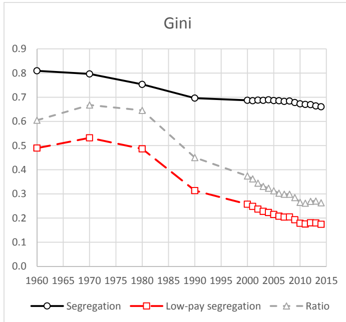
b: Gini
