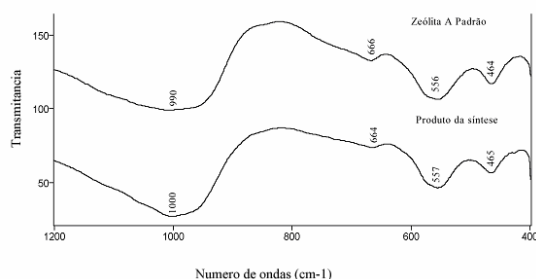
Figura 6. Espectros vibracionais das amostras de zeólita padrão A e do produto da síntese.
