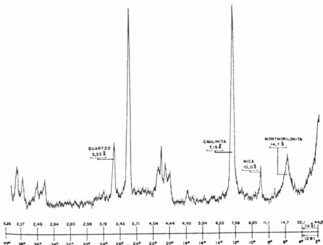
Figura 2. Difratoograma de raios X de uma mistura artificial de caulinita (70%), montmorilonita (10%), mica ou illita (5%) e quartzo (5%). (Santos, 1975).
