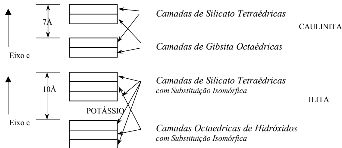
Figura 1. Esquema da distância interplanar da caulinita e da ilita (Santos, 1975).
