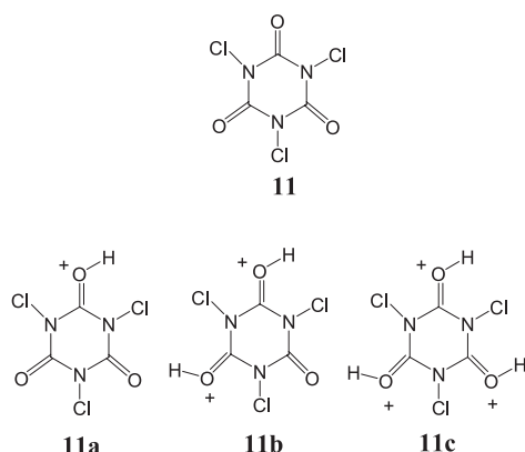
Figura 2. Espécies supereletrofílicas ( 11a , 11b e 11c ) formadas da reação entre ATCI e H_2SO_4
