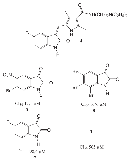
Figura 1. Estrutura do sunitinibe (4) e dos derivados da isatina nitrados e halogenados (5-7) acompanhados dos seus respectivos valores de Cl_{50}
