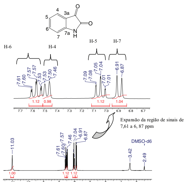
Figura 4. Espectro de RMN ^1\text{H} da isatina
