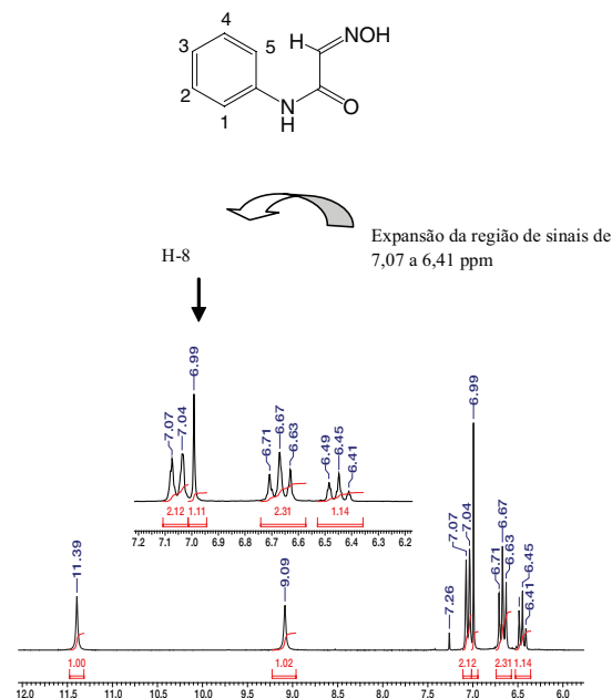
Figura 3. Espectro de RMN ^1H da isonitrosoacetanilida
