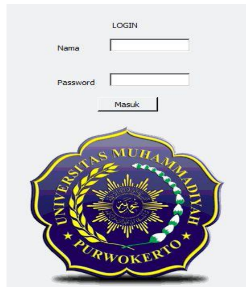
Gambar 4. Halaman Login
