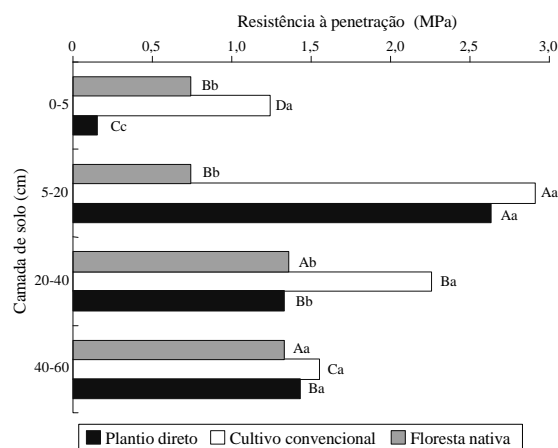
FIG. 2. Resistência à penetração em diferentes camadas do Latossolo Roxo, nos sistemas plantio direto, cultivo convencional e floresta nativa. Médias com a mesma letra, maiúscula (comparação entre sistemas de manejo) e minúscula (comparação entre sistemas de manejo dentro de cada profundidade), não diferem entre si a 5% de probabilidade pelo teste de Tukey.
