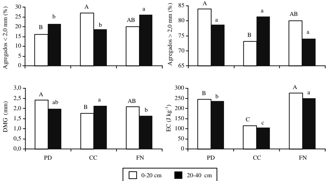
FIG. 1. Distribuição, diâmetro médio geométrico (DMG) dos agregados e energia cinética (EC) necessária para destruir os agregados, nos sistemas plantio direto (PD), cultivo convencional (CC) e floresta nativa (FN) em Latossolo Roxo. Médias com a mesma letra, maiúscula na camada superficial e minúscula na camada subsuperficial, não diferem entre si a 5% de probabilidade pelo teste de Tukey.
