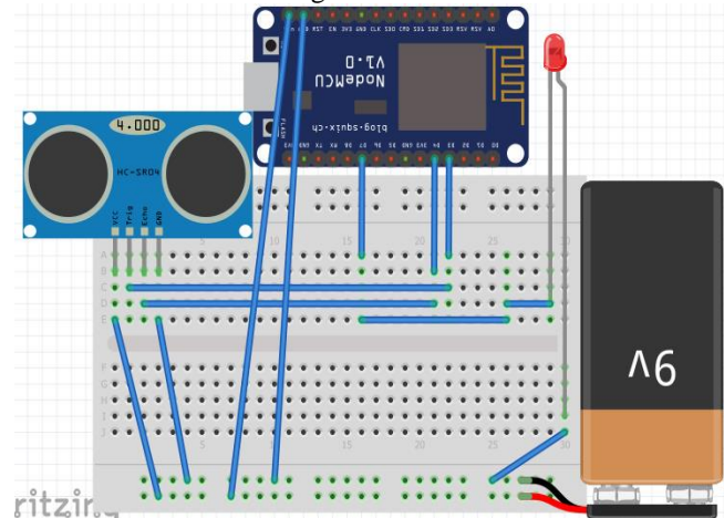
Figure5: Smart pendant
