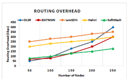
a) Scenario 01 (10%SDN hybrid nodes + 90%Legacy nodes)
