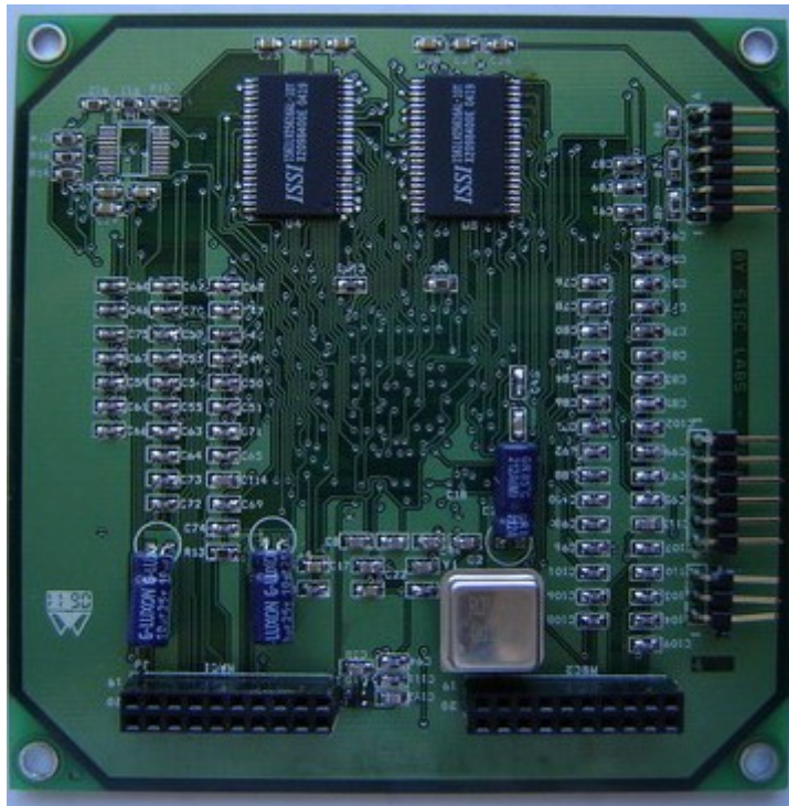
Ilustração 7.13.1.2: Vista do verso da placa desenvolvida.
