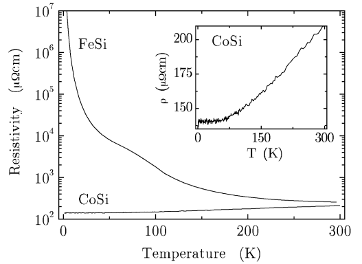
Fig. 6. Resistivity of FeSi and CoSi.
