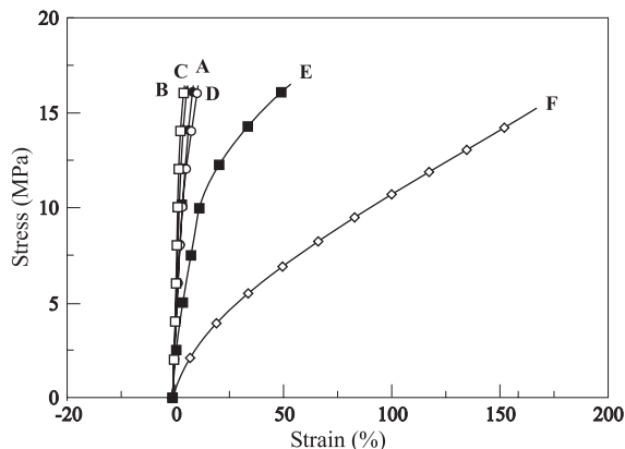
Figure 8. Stress-strain curves of Nafion- \text{Cs}^+ membranes at different temperatures: (A) (—●—) room temperature; (B) (—□—) 60°C; (C) (—▲—) 90°C; (D) (—○—) 120°C; (E) (—■—) 150°C; and (F) (—◇—) 180°C
