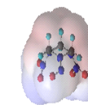
2 MONORDX
