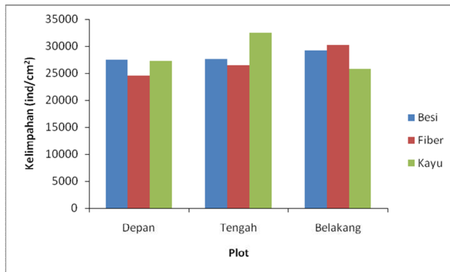
Gambar 4. Histogram Rata rata Kelimpahan Diatom Epilitik pada Kapal Kayu, Besi dan Fiber
