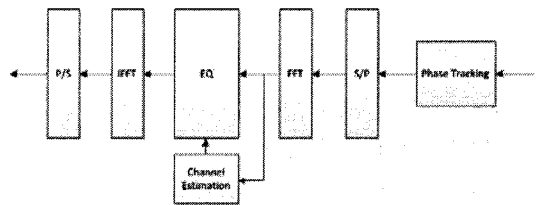
(a) SC-FDE 시스템의 시간 영역 위상 추적 블록도 (FDE 이전 추적 블록)
