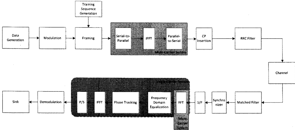
그림 2. SC-FDE 시스템 블록도 - FDE를 갖는 단일/다중 반송과 시스템 비교 (제안 위상 추적 포함)
