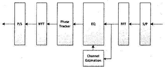
(d) 제안하는 SC-FDE 시스템의 주파수 영역 위상 추적 블록도 (주파수 영역 위상 추적)
