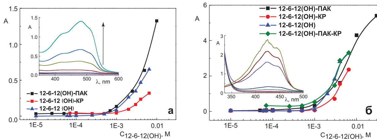
Рисунок 4. Зависимость оптической плотности Судана I (а) и куркумина (б) при 495 и 427 нм соответственно, от концентрации ПАВ в индивидуальной, бинарной и тройной системах; C_{\text{ПАК}}=1 мМ, 25 °С. На вставках спектры поглощения Судана I (а) и куркумина (б), 25 °С, l=0.2 см.
