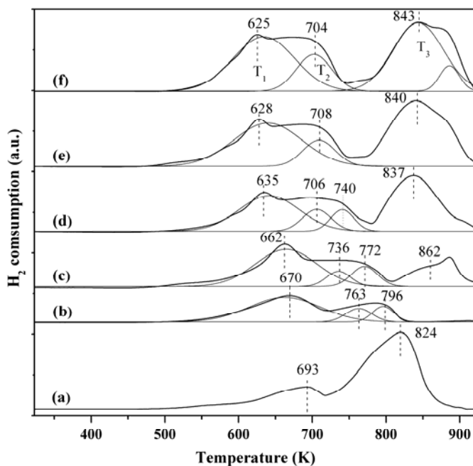
Figure 7. \text{H}_2 -TPR profiles of the catalysts \text{Mn-Co/TiO}_2 (773 K) with various Co contents: (a) 5\text{Co/TiO}_2 ; (b) 10\text{Mn/TiO}_2 ; (c) 10\text{Mn-2Co/TiO}_2 ; (d) 10\text{Mn-5Co/TiO}_2 ; (e) 10\text{Mn-8Co/TiO}_2 ; and (f) 10\text{Mn-10Co/TiO}_2 .
