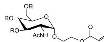
M118a , R = H M118b , R = SO 3 - Na +
