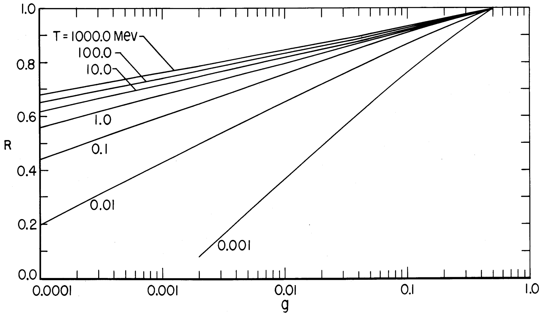
a. Electrons: g \leq 0.5
