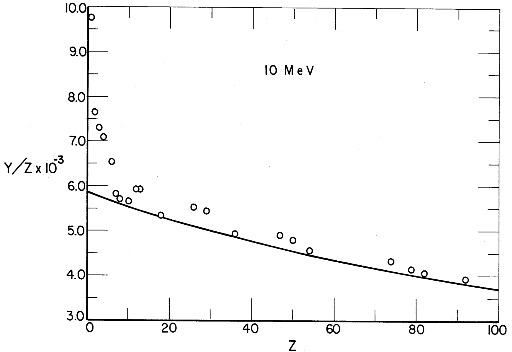
a. 10 MeV
