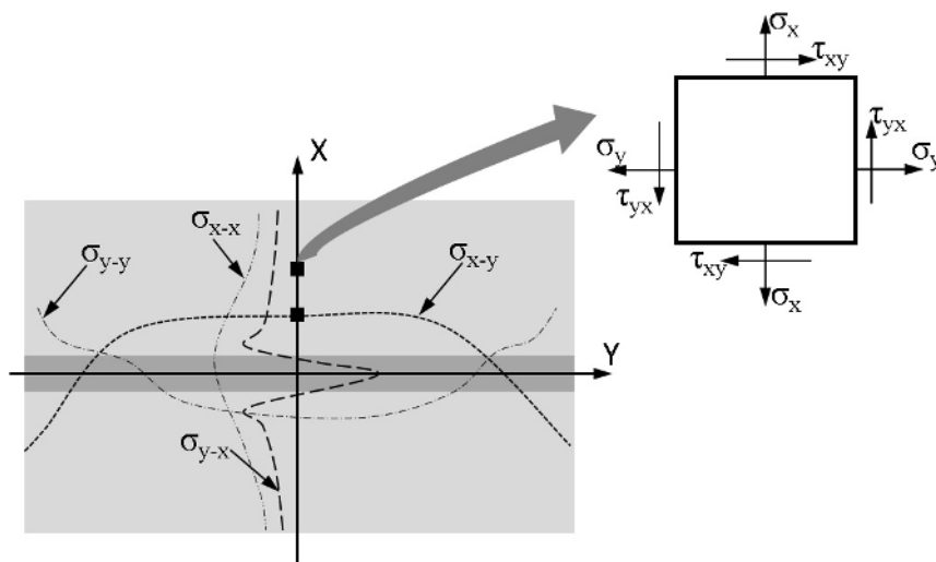
Figura 2. Esquematização de distribuição das TR em um plano sobre uma chapa soldada e representação proposta pelos autores para cada componente das tensões. Fonte: Elaborada pelos autores.
