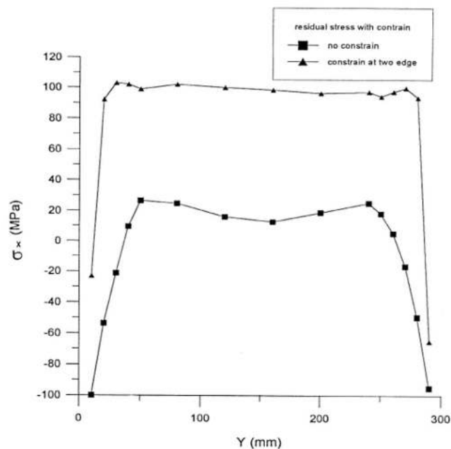
Figura 9. Distribuição de TR transversais em função da restrição da chapa de teste (Teng e Lin, 1998).
