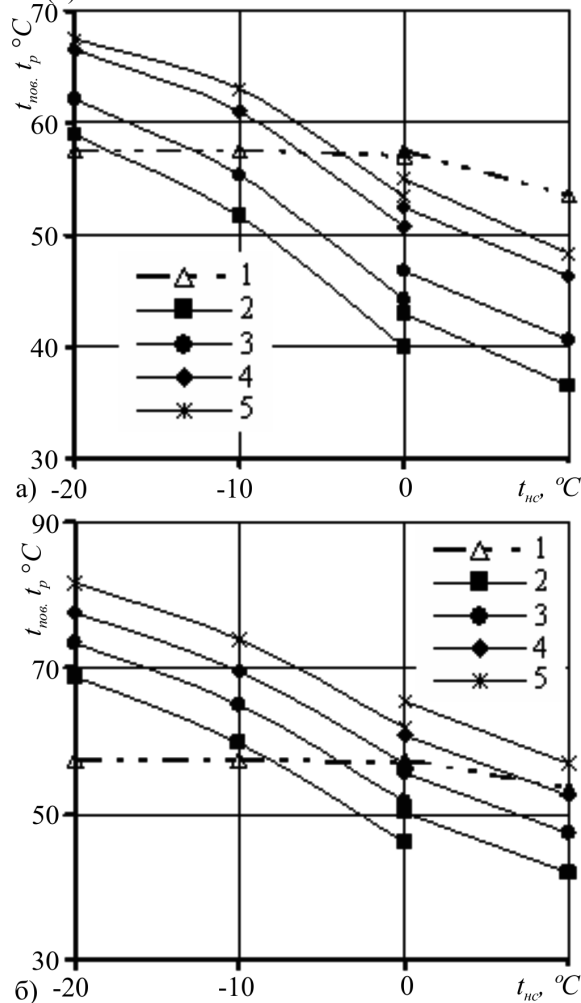
Рис. 3. Залежність температури внутрішньої поверхні t_{нов} в усій димові труби (2-5) і точки роси t_p (1) від температури навколишнього середовища t_{nc} для залізобетонних димових труб та різних часток байпасування \chi : а) без футерування; б) з футеруванням; 1 – t_p ; 2 – \chi = 0\% ; 3 – 10%; 4 – 20%; 5 – 30%
