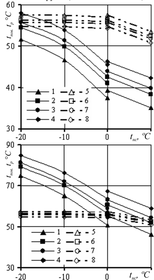
Рис. 4. Залежність температури внутрішньої поверхні t_{нов} в усій димові труби (1-4) і точки роси t_p (5-8) від температури навколишнього середовища t_{nc} за t_{zn} = 150^\circ\text{C} , t_{zn} = 160^\circ\text{C} за різних часток підмішаного повітря \sigma : 1, 5 – \sigma = 0\% ; 2, 6 – 8%; 3, 7 – 12%; 4, 8 – 20%; а) металеві; б) цегляні димові труби
