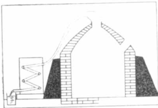
Abb. 2. Querschnitt der Destillationsanlage.
