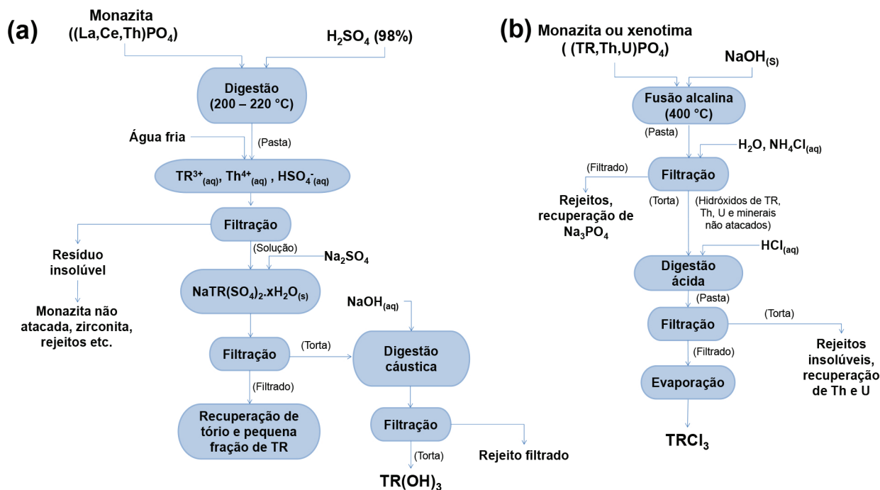
Figura 13. Esquematização das metodologias de processamento da monazita e xenotima através (a) de abertura ácida por ataque com ácido sulfúrico e (b) abertura alcalina utilizando-se soda cáustica (Reproduzido da Ref. 1)
