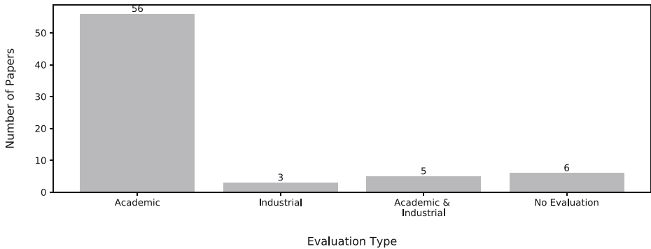
Fig. 14 Evaluation Type
