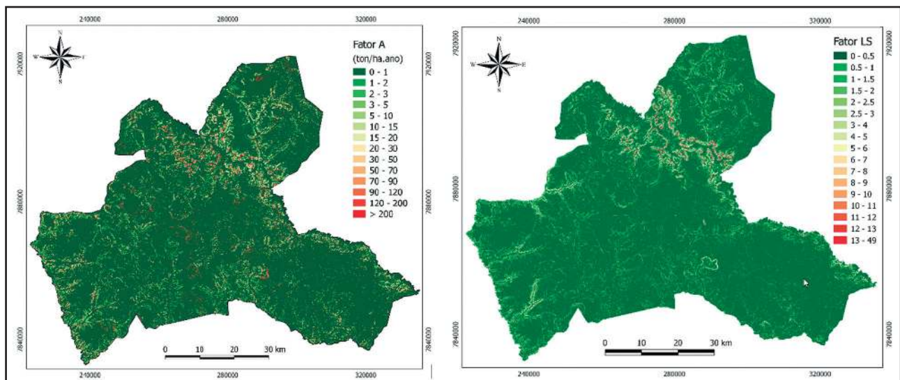
Figura 8 Comparação entre o mapa do Fator A, perda de solo por erosão laminar e o mapa do Fator topográfico (LS).
