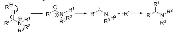
Scheme 1.4
