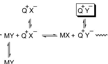
Brändström–Montanari Modification
