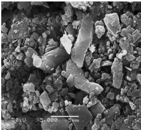
Рис. 16. Структура забрудненого цементного каменю залізобетонних шпал
