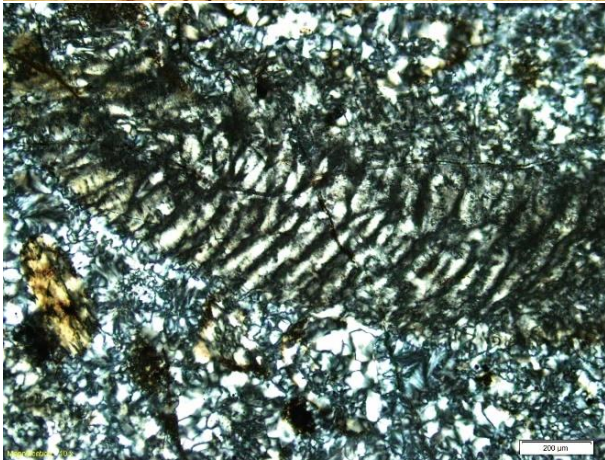
SO-05: Bioclasto silicificado conservando su estructura interna original.
