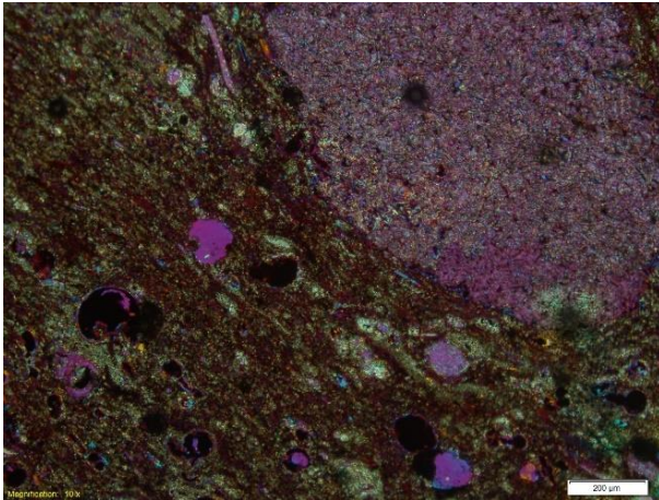
SO-16: Bioclastos rellenos de hidrocarburo y concreción calcárea
