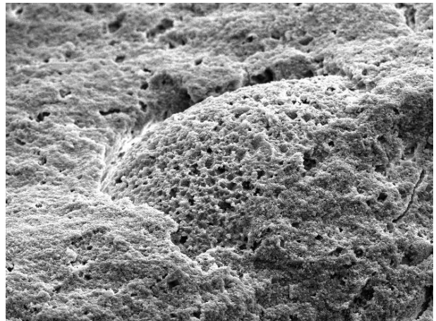
SP-1802: Porosidad secundaria intercrystalina
