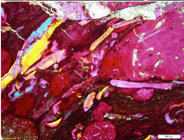
SA-1909: Bioclastos fosfáticos de fluorapatito.
