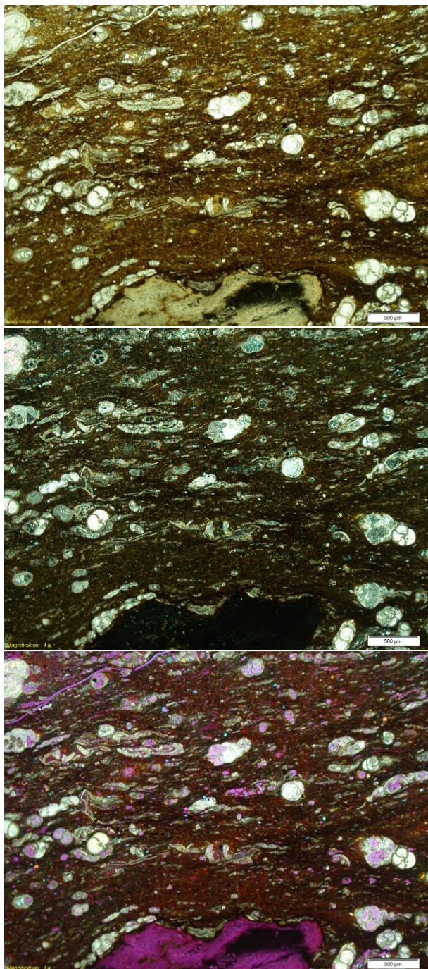
SA-1936A: Laminación deformada alrededor de peloide.
