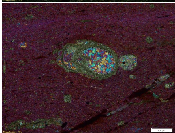
SA-1930: Foraminífero relleno de cuarzo con remplazamiento en su caparazón, en medio de matriz totalmente silicificada.
