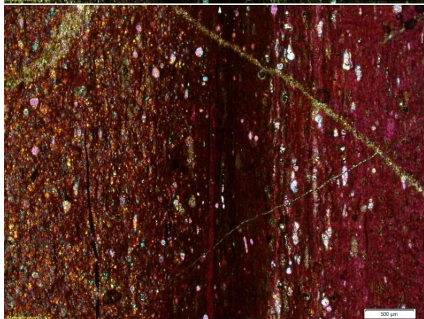
SO-32: Lamina rica en materia orgánica separando diferentes tamaños de silicificación en la matriz
