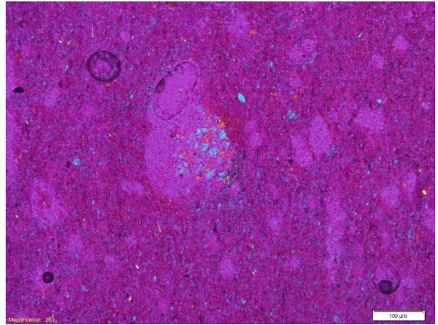
SF-1802: Relleno de cuarzo en molde de foraminífero.
