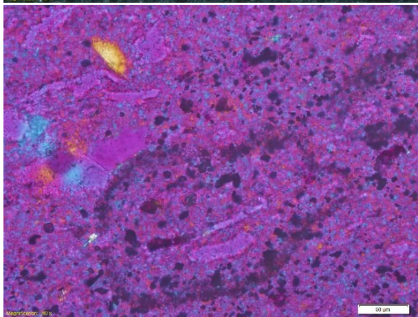
SP-1801: Moldes de foraminíferos en medio de matriz totalmente silicificada.
