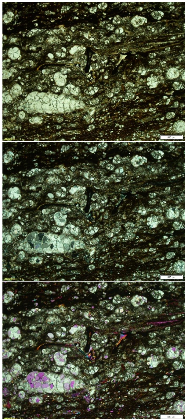
SA-1938: Foraminíferos bentónicos rellenos de calcita y restos óseos fosfáticos
