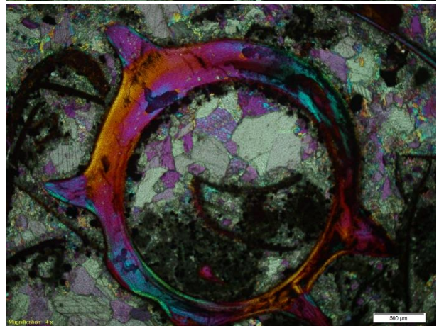
SA-1915: Vertebra de pez compuesta de fluorapatito con estructura geopetal.
