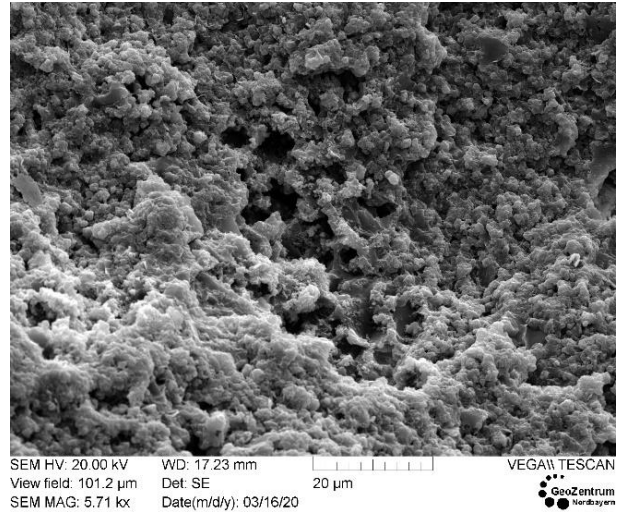
SA-1930: Textura euhedral en contacto puntual
