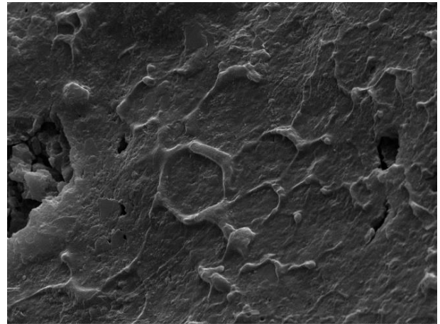
SA-1936: Marcas de cemento a través de cristales hex
