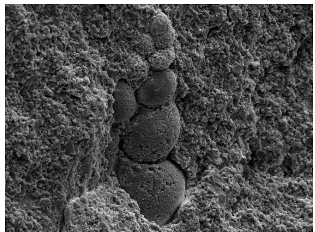
SA-1936: Textura de matriz rodeando relleno de for.
