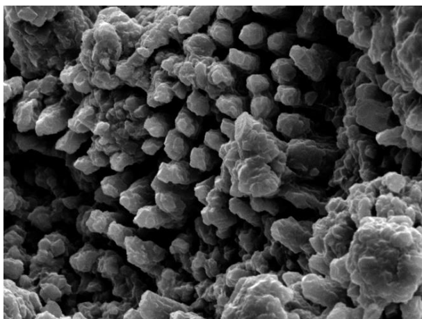
SA-1933: Rellenos de cámaras de foraminíferos.
