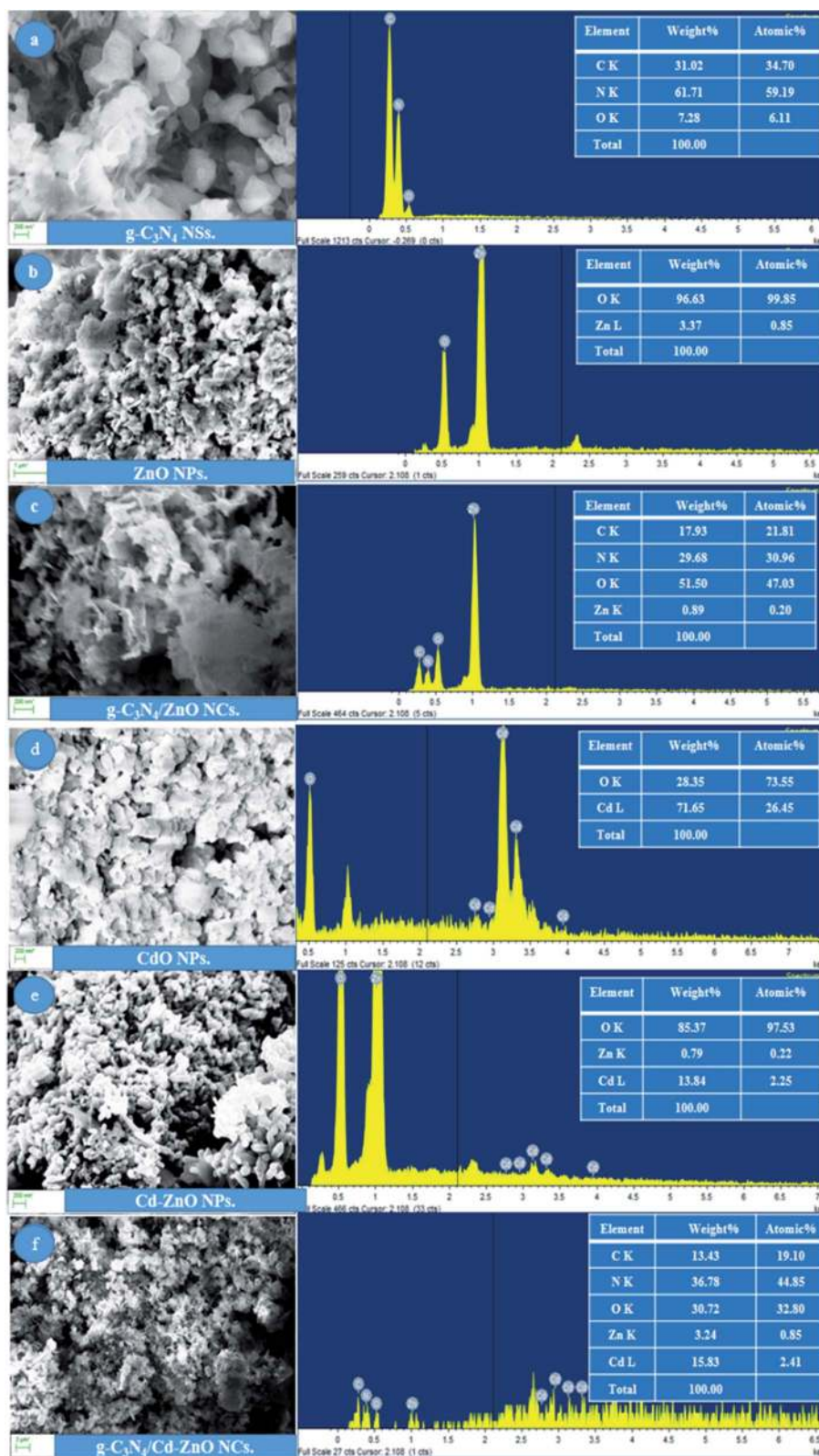
Fig. 2 SEM images and EDS spectra of (a) g-C 3 N 4 NSS, (b) ZnO NPs, (c) g-C 3 N 4 /ZnO NCs, (d) CdO NPs, (e) Cd-ZnO NPs, and (f) g-C 3 N 4 /Cd-ZnO NCs.
