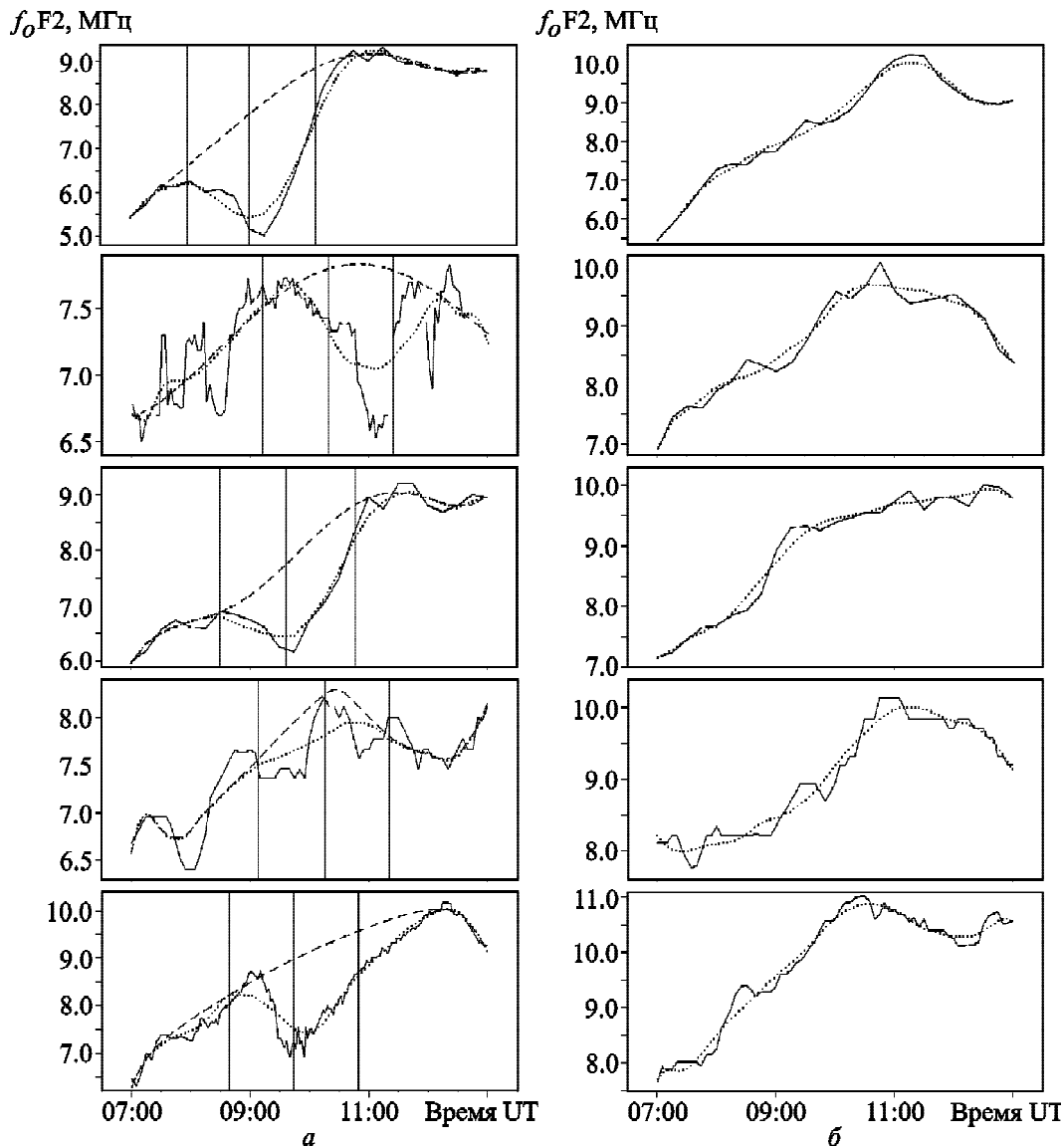
Рис. 3. Временные зависимости критической частоты (сплошная линия) и сглаженной скользящим средним критической частоты (пунктирная линия) для ионозондов (панели сверху вниз) El Aginosillo, Москва, San Vito, Харьков, Athens: а – 20 марта 2015 г., б – 21 марта 2015 г. Штриховая линия описывает ожидаемые вариации f_oF2(t) в отсутствие СЗ
