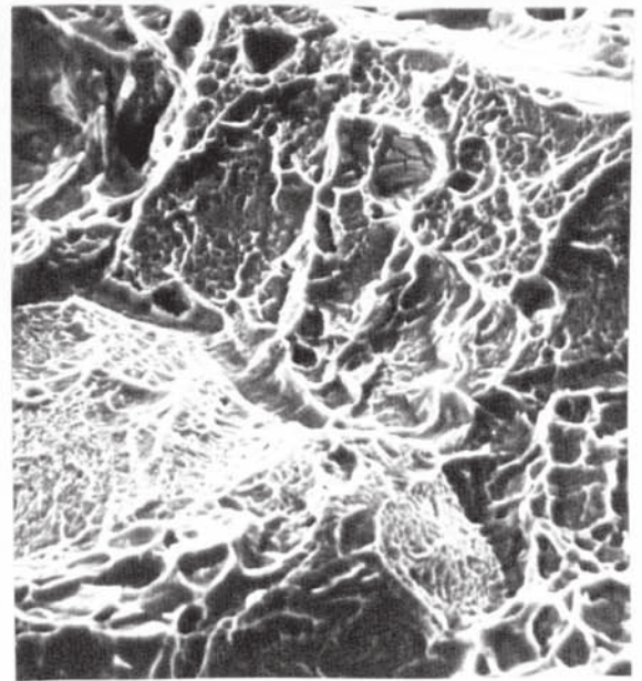
(d) Inclusions in flatter "intergranular" fracture. 1300°C+
