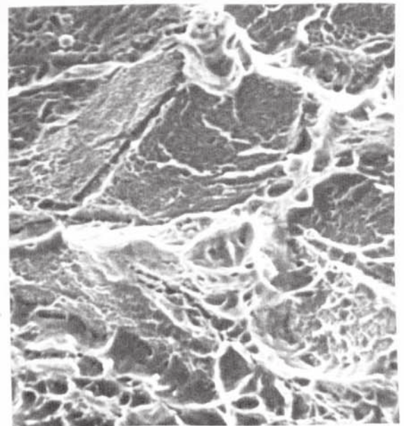
(d) Fracture adjacent to the fusion boundary. 1400°C+
