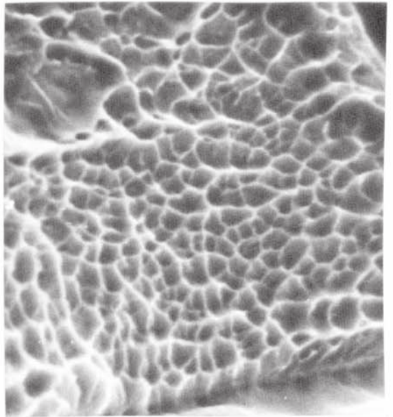
(d) Dimples in(c). x 7000
