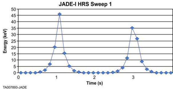
Fig. 74 One JADE-I HRS ESA sweep
