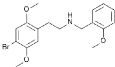
25B-N-BOMe
