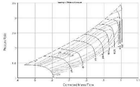
Fig. 7. 저압압축기 성능선도
