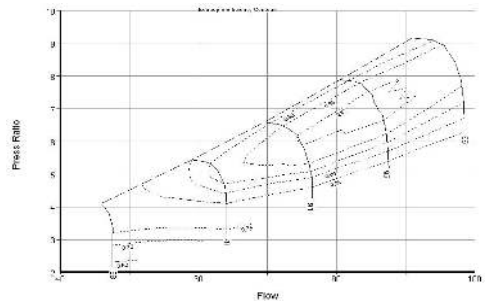
Fig. 8. 고압압축기 성능선도
