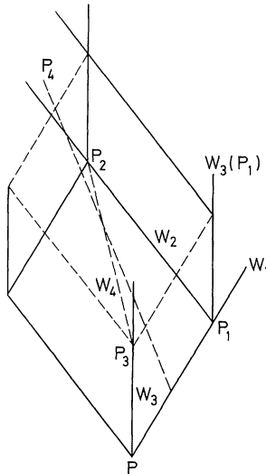
Fig. 1. Proof of Lemma 3.2
