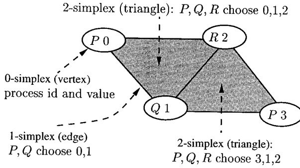
FIG. 4. Vertexes and simplexes.
